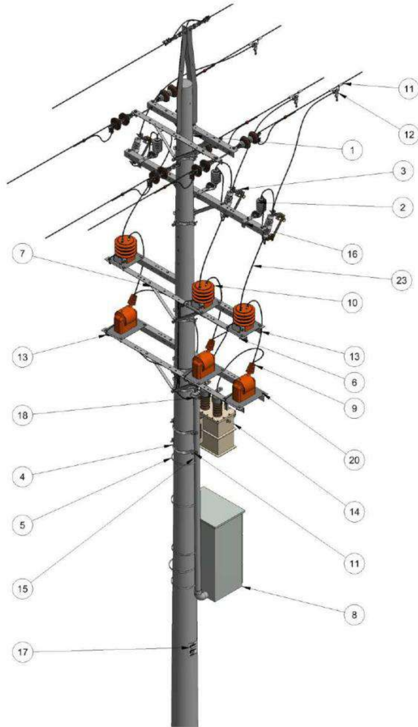
Figura 8. Montaje trifásico disposición cruceta al centro. Vista Isométrica
