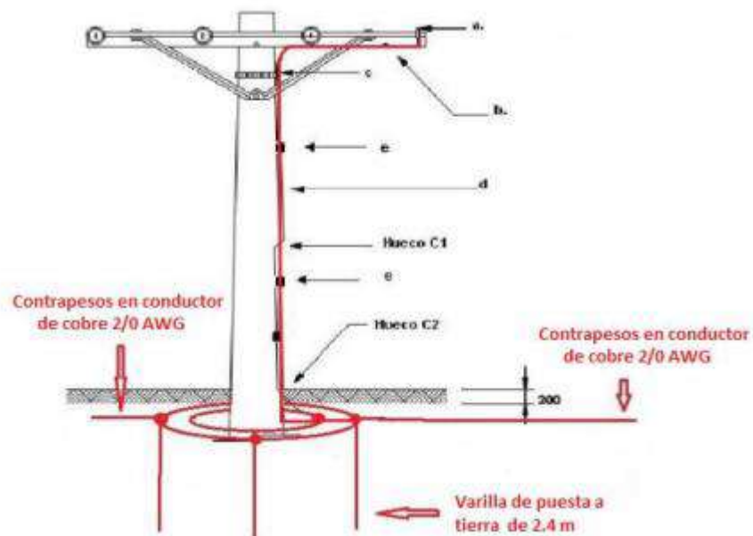
Figura 3. Sistema de puesta a tierra de referencia, incluyen el uso de contrapesos.
