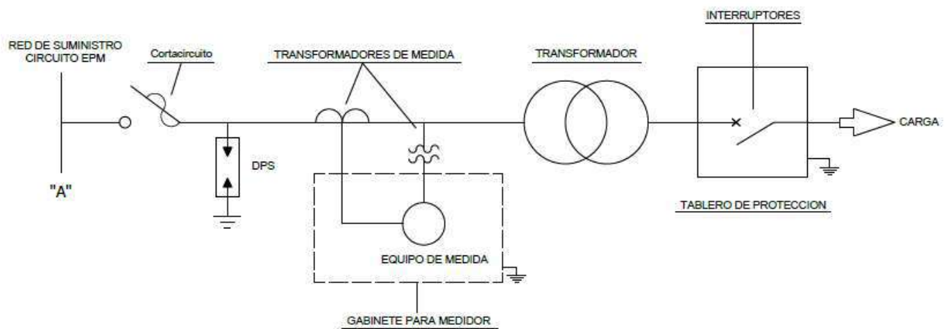
Figura 1. Diagrama unifilar ubicación de sistema de medida en instalaciones con transformadores de distribución de potencia monousuario definidos como activos de conexión
