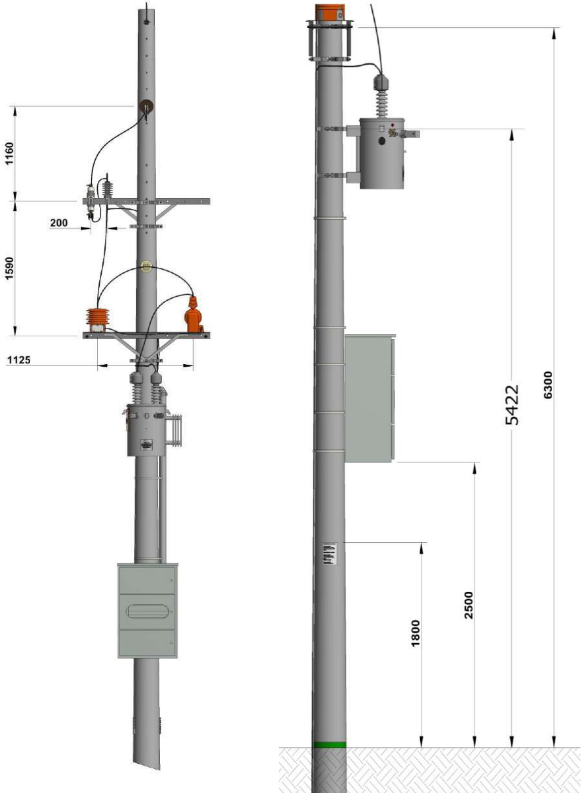
Figura 5. Montaje monofásico disposición cruceta al centro. Vista frontal y lateral
