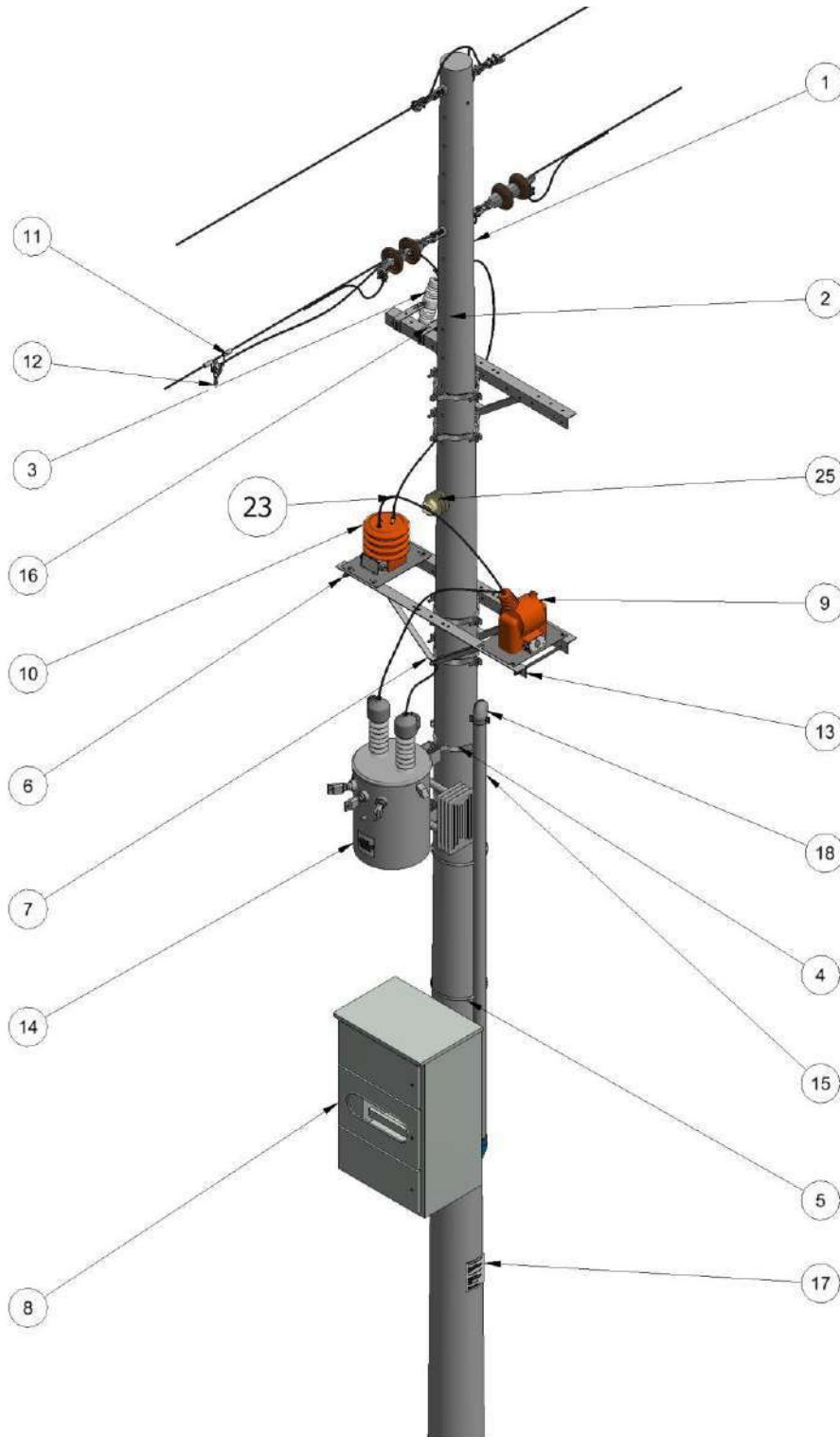
Figura 4. Montaje monofásico disposición cruceta al centro. Vista Isométrica
